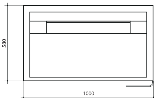
Vezérlőpanel (IQ-32)
